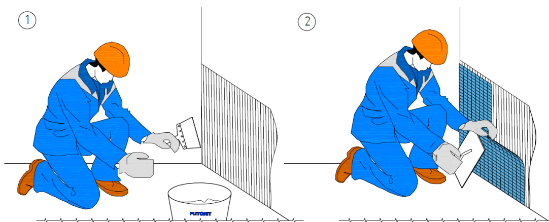
Рис. 23. Организация работ по приклеиванию мозаики
