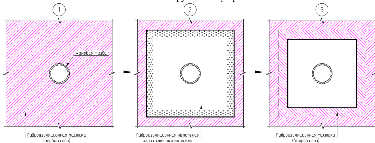
Рис.18.4. Последовательность нанесения гидроизоляционной манжеты.
