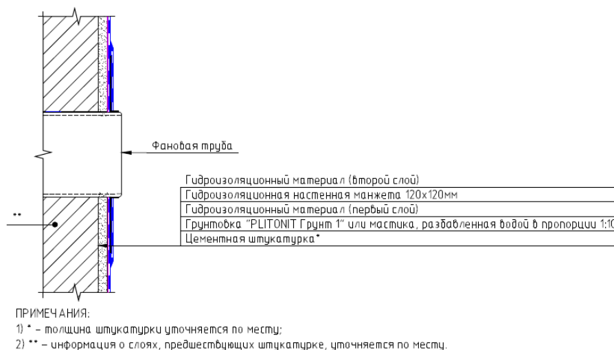
Рис.18.2. Конструктивный разрез №2.
