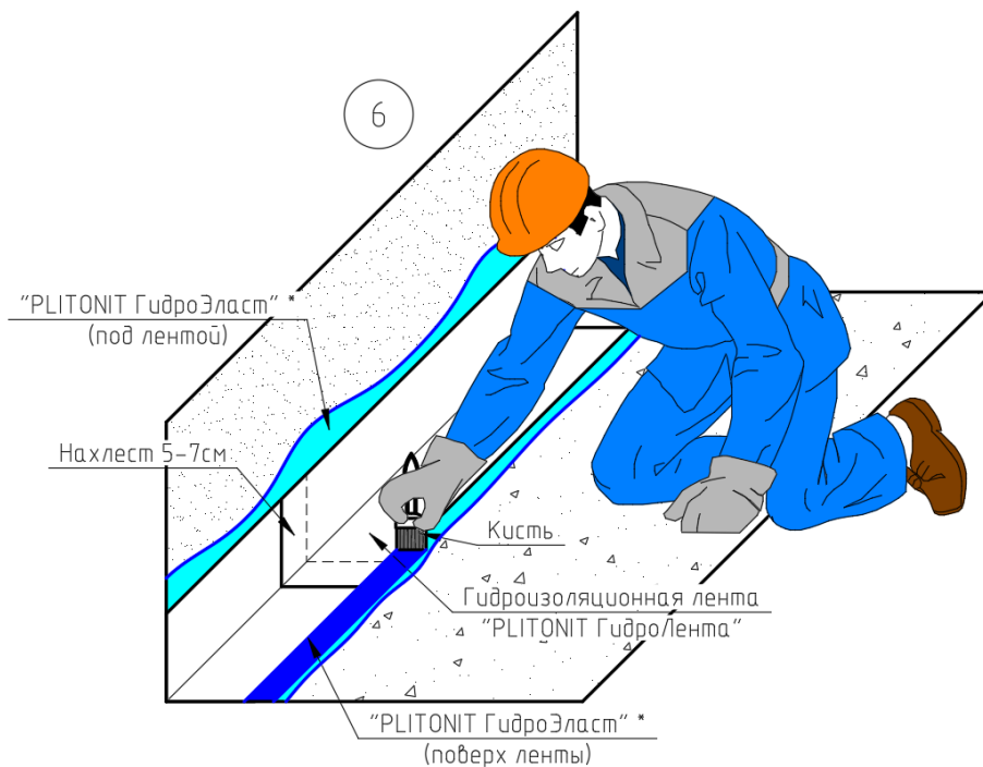
Рис.19.1. Последовательность работ (на стенах работа в аналогичном порядке), где: 1 - проверка ровности основания контрольной рейкой (аналогично для горизонтальной поверхности); 2 – размешивание емкости с мастикой; 3 – нанесение первого слоя мастики, разбавленной водой в пропорции 1:10, на основание; 4 – нанесение гидроизоляции на поверхность (аналогично для горизонтальной поверхности); 5 – укладка гидроизоляционной ленты на поверхность, предварительно обработанную «PLITONIT ГидроЭласт» или «PLITONIT WaterProof Standard»; 6 – поверхностная обработка ленты мастикой «PLITONIT ГидроЭласт» или «PLITONIT WaterProof Standard».
