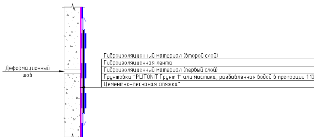
Рис.18.3. Конструктивный разрез №3.
