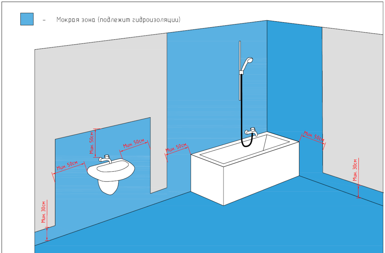
Рис. 19.2 Мокрые зоны внутри влажных помещений, подлежащие гидроизоляции.
